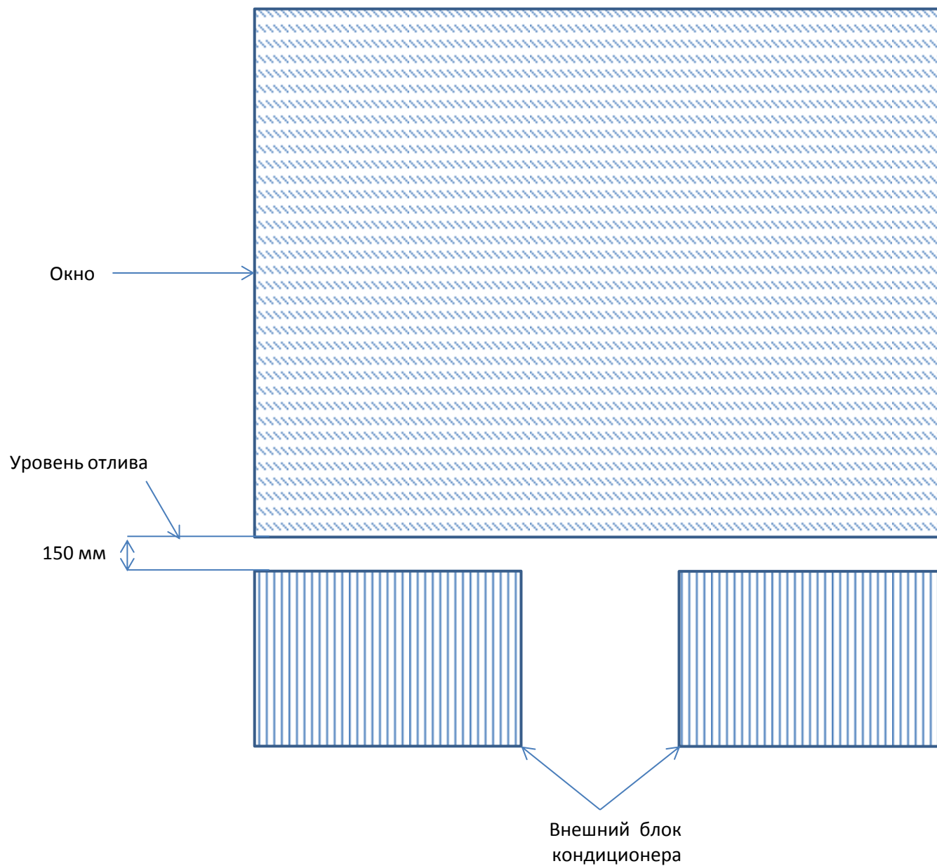
Схема монтажа внешнего блока Системы на фасад здания (под окно). Вид спереди.
